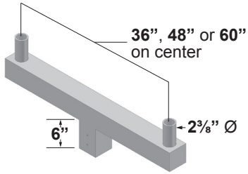
SCA-2 EPA 36"-1.8 / 48"-2.3 / 60"-2.7
