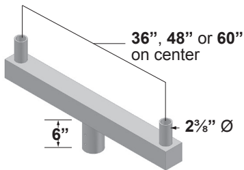
RCA-2 EPA 36" - 1.8 / 48" - 2.3 / 60" - 2.7
